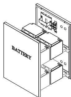
8pcs Batteries 38AH/45AH 198 × 166 × 170 (L × W × H)
